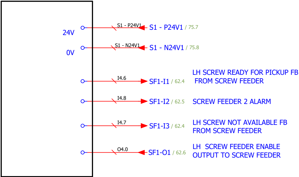
DEPRAG Mini Screw Feeder_189x103x156
